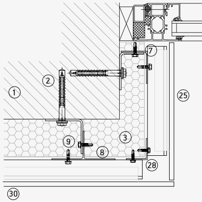
Dekton jamb
