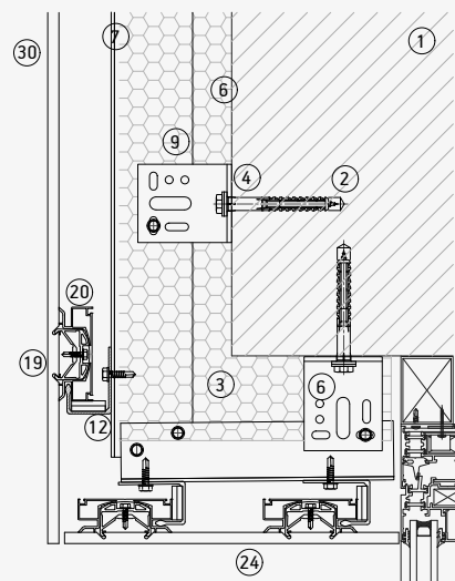
Dekton lintel
