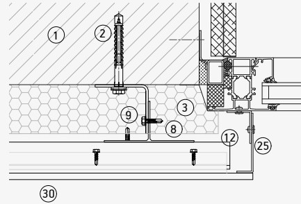
Metallic jamb
