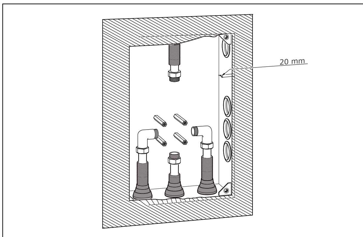
4.1 Självhäftande tätband fästes på vägg och viks ner minst 20 mm i boxen.
