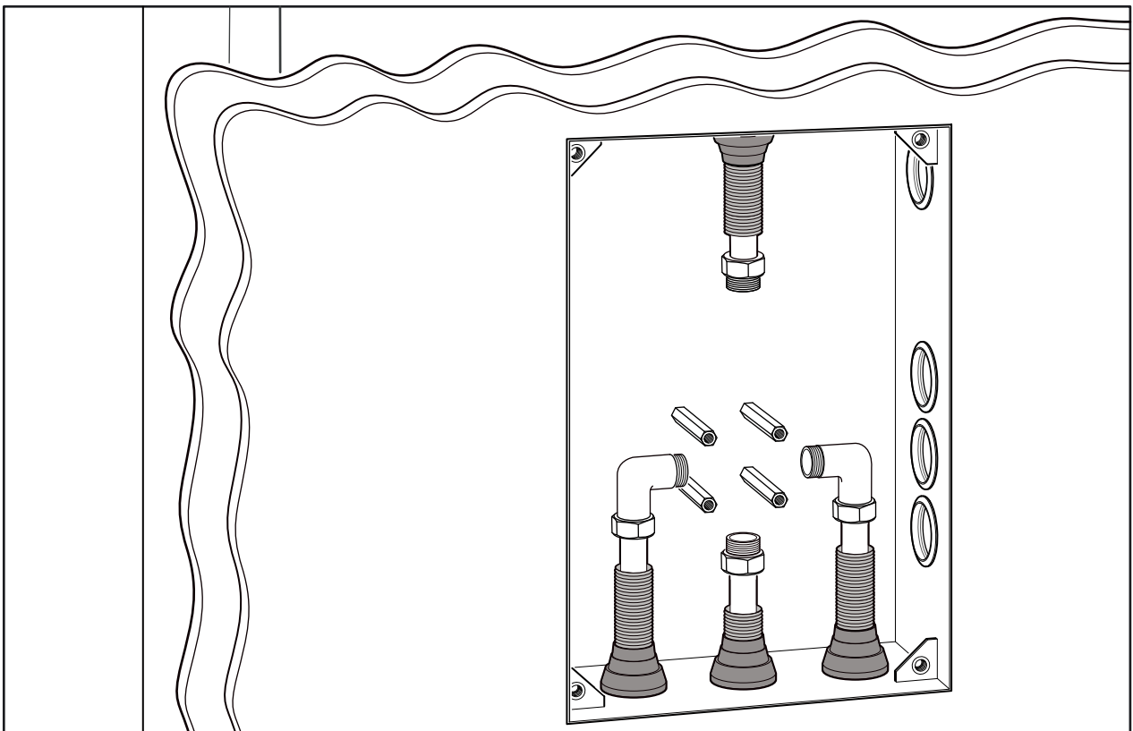
2.7 Väggsnivåerna monteras av byggtreprenören och ska ansluta mot boxens ytterkanter. Tätskikt appliceras enligt anvisningar i avsnitt 4.
