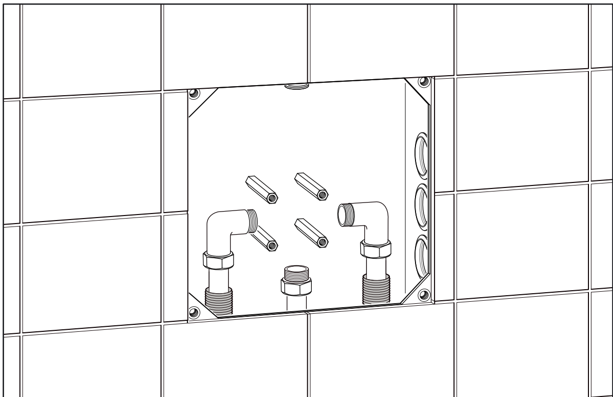
4.3 Väggytskiktet av keramiska plattor monteras. Urtaget för blandarbrickan ska göras till jäms med teleskopdelens hålkantar. OBS att skruvhålen för blandarbrickan inte ska täckas av kaklet och att gängorna ska skyddas mot intrång av fästmassa.
