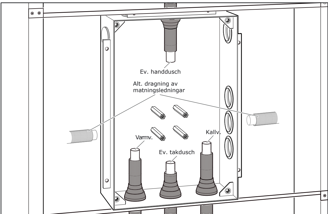
2.5 De anslutande rörledningarna dras in i Boxen och längdanpassas.
